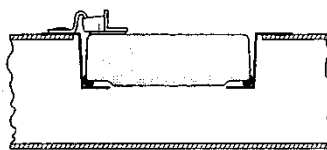
Einbau innen im Kanal (nicht isolierte Kanäle)
