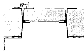
Einbau aussen am Kanal (50 mm dicke Isolierung und Distanzrahmen)
